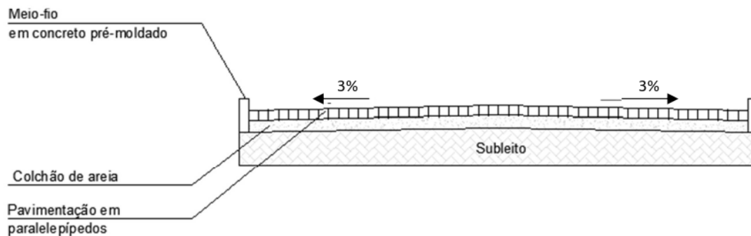
Figura 5 - Seção típica para ruas
