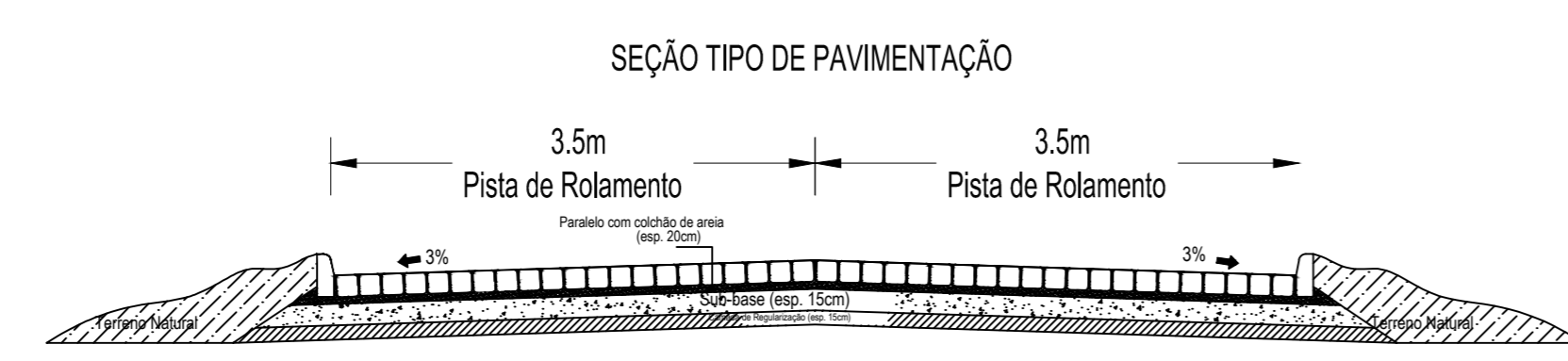
Seção Transversal Tipo Escala: 1/100
