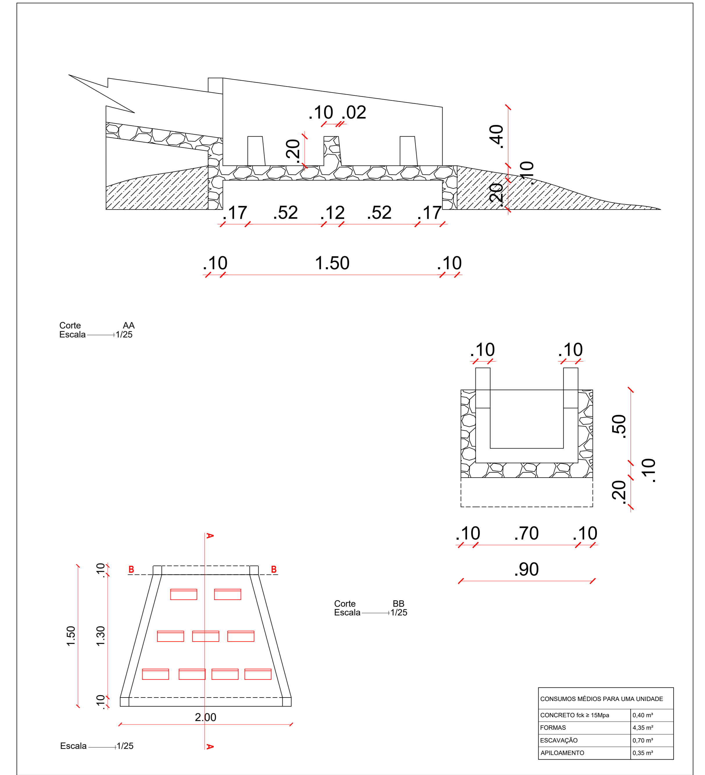
Detalhe Dispositivo de Drenagem - Dissipador de Energia - DED - 01
